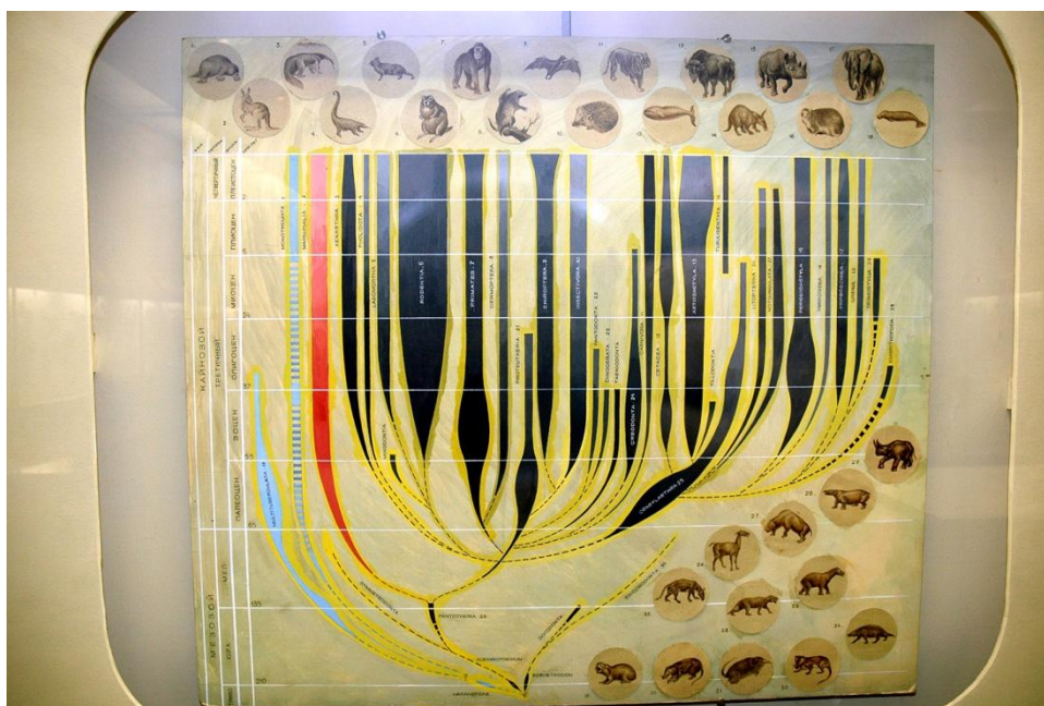
Рис.25. Отсутствие останков предков млекопитающих
