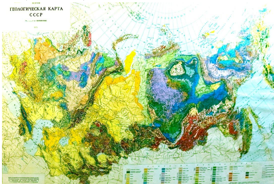
Рис.2. Геологическая карта СССР.
