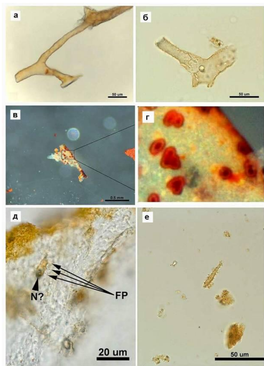
Рис.32 Останки мягких тканей и клеток в бедренной кости тиранозавра
