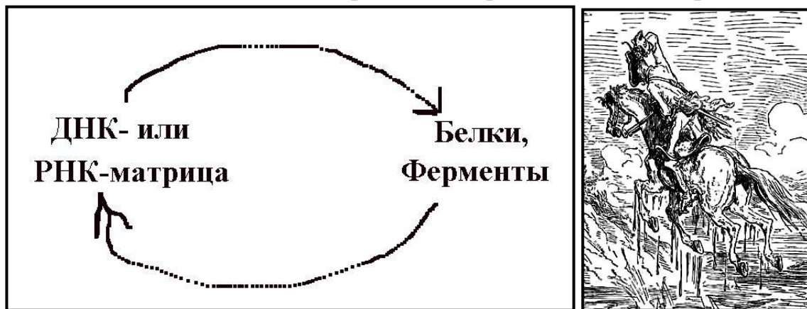
Рисунок 5. Нерешаемая проблема абиогенеза: замкнутый круг. ДНК или РНК матрицы не могут существовать без сложнейших белков и ферментов их репарации, а последние не могут кодироваться ничем иным, кроме как ДНК (или РНК). Решение этой проблемы — сродни вытаскиванию бароном Мюнхгаузенем самого себя за волосы из болота.
