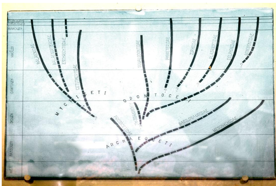
Рис.26. Отсутствие предков китообразных
